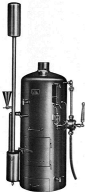
Typ F 120 med förvärmare och pump.
