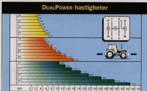
En enkel knapptryckning reducerar arbetshastigheten med 18% och ökar vridmomentet till hjulen med 22%. Ett exempel på DUALPOWER systemets fördelar i din Serie 40 SL traktor.
