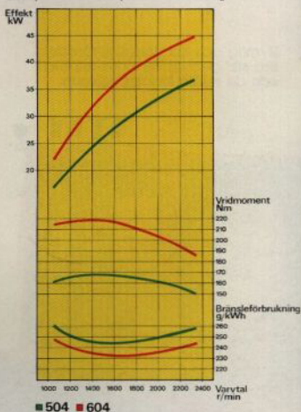
Effekt, vridmoment och spec.bränsleförbrukning
