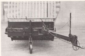
Vagnar med typbeteckningen LL-S är utrustade med rullgrat svängdrag och extra ramförstärkning. Pick-uplyften manövreras med lindrag. (Levereras endast efter överenskommelse.)
