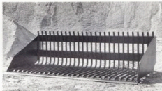
Stengrep med raka pinnar och skärstål för hjullastare. Användes ex.vis vid upplastning av torv vid kantskäring av vägrenar, uppbyggnad och lastning av gatsten.
