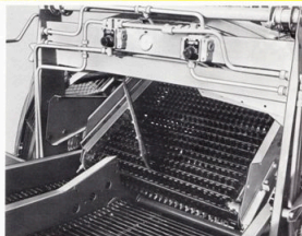
○ Bakåtgående gummifingerband för mycket lätta, stenfria jordar (lagerföres ej).
