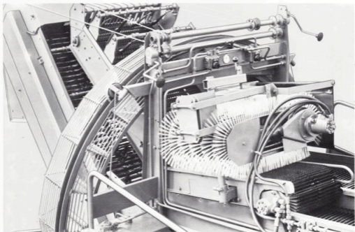
Hydrauldrivet stenfrånskilningsaggregat med reglage.
