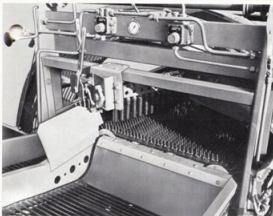
○ Tvärgående gummifingerbandet med pendelkam, speciellt för kokbildande jordar.
