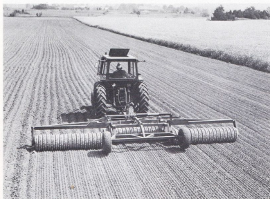
Vågig ring för effektivare jordbearbetning.
