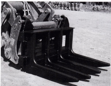
Stenbrytare för hjullastare. Avsedd för uppbyggnad och borttransport av stor sten, stubbar m. m.
