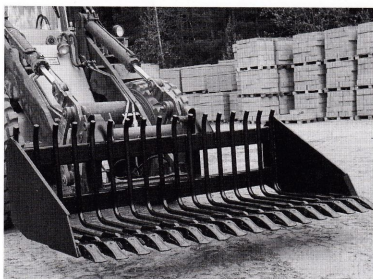
Stengrep med holtkänder för hjullastare. Användes exempelvis vid byggande av skogsbilvägar och olika krävande sorteringsarbeten.
