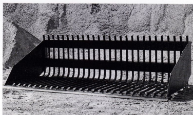
Stengrep med raka pinnar och skärstål för hjullastare. Användes exempelvis vid upplastning av torv vid kantskärmning av vägrenar, uppbyggnad och lastning av gatsten.
