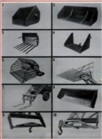
För ALÖ-Quicks finns 10 olika utrustningar med anslutningsring, extern koppling och berging med hjälp av reorutrustning.
