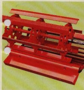
Tröskcylinder och slagsko
