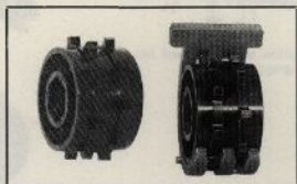
Standard- och småfrövals. Till standardvalsens kan en reducerare erhållas (se bilden).
