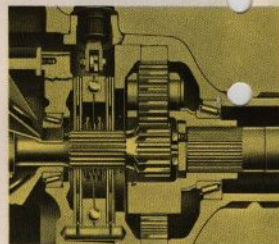
Helkapslade skivbromsar
