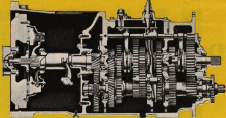
Ny växellåda
