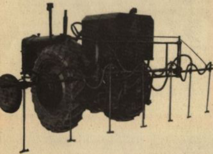
Vätskespridare för bekämpning av ogräs och insekter. Behållaren rymmer 450 liter, arbetsbredd 7 rader. Pumptryck 15 kg.
