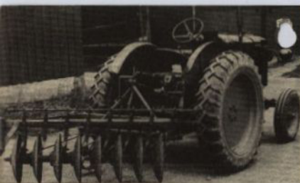
Tallriksskumplog (Lilla Harrie) för stubbearbetning.
