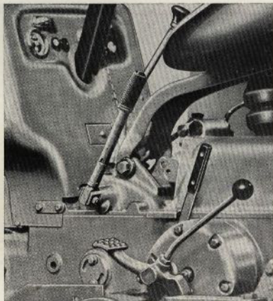
Denna bild visar den teleskopiska AGRIOMATIC-spaken, som har enkel-skift. Fot- och handmanövrerad differentialspärr, som kopplar ur automatiskt.
