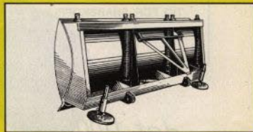
SCHAKTBLAD. Bredd 2,4 meter. Ställbart 30°. Ställbara stöd tallrikar. Utbytbar slättstål. Fjäderbelastad utlösningsmekanism.
