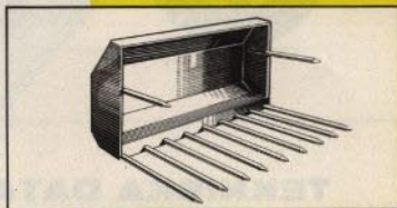
GÜDELGREP. Bredd 1,5 meter. Tolv specialhårdade pinnar.
