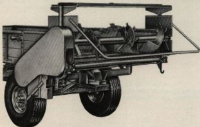
VESTAS som stallgödselspridare. Av- och påmontering av aggregatet kan ske på några minuter.
