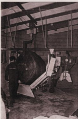
Balen lyfts i med en eltelfer som hänger i en tvärgående balk.
