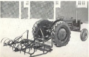
En 15-pinnars hydraulburen sladdfjäderharv ger bekväm bearbetning ända ut i besvärliga böm.
