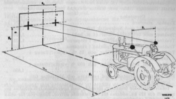
Bild 34. Inställning av strålkastarna.
