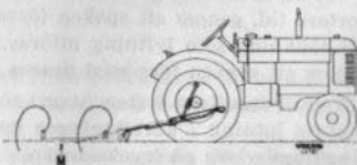
Bild 10. Dragbommens inställning — sladdfjäderharv.
