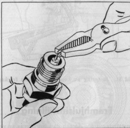
Bild 30. Justering av tändstiftens gnistgap.
