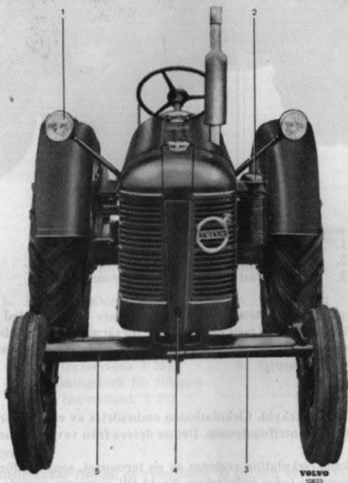
Bild 21. Traktorn framifrån.
