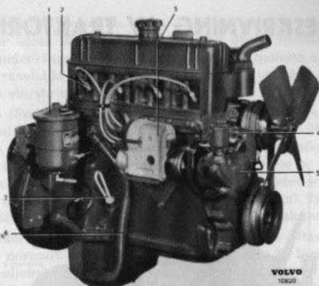
Bild 17. Motorn från höger.
