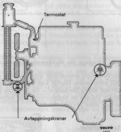
Bild 28. Kylsystemets avtappningskranar.
