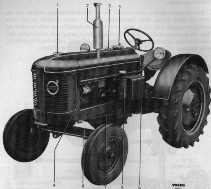
Bild 19. Traktorn från vänster.
