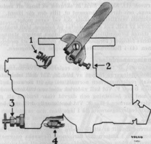
Bild 25. Förgasarinställning.
