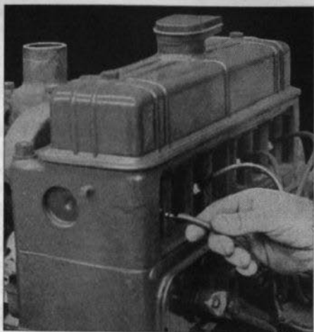
Bild 37. Provning av tändningssystemet.
