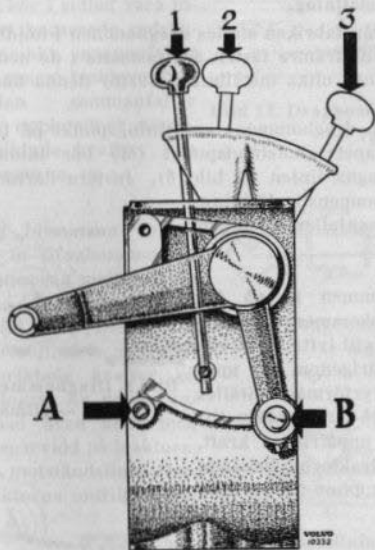
Bild 7. Manöverspak för hydraulisk lyft.
