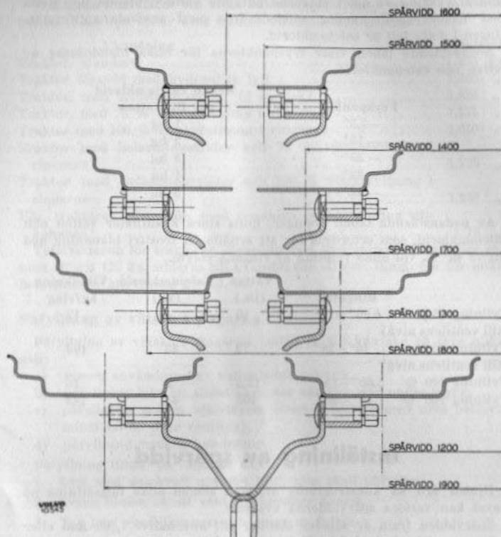
Bild 35. Inställning av spårvidden.
