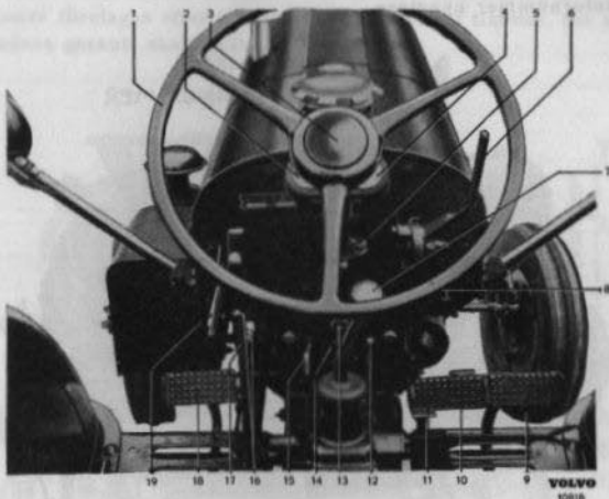
Bild 2. Instrument och manöverorgan.
