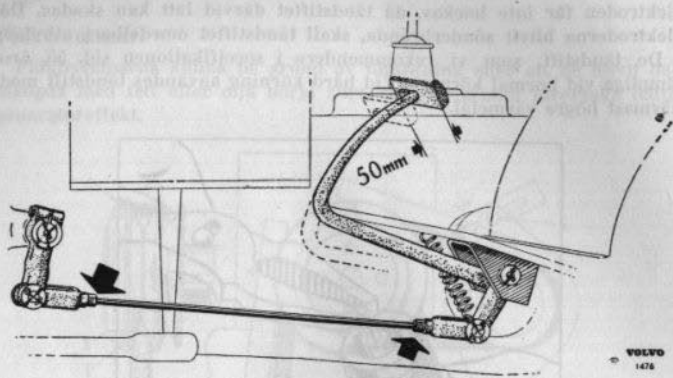
Bild 31. Justering av kopplingspedalens frigång.
