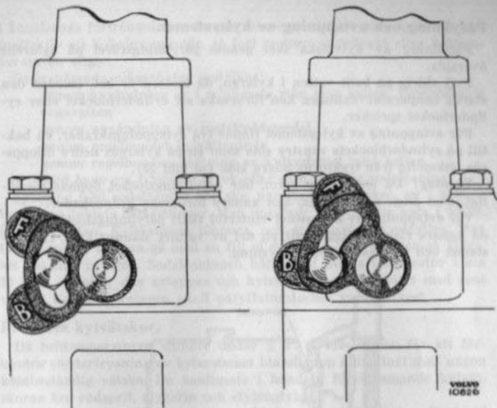
Bild 26. Reglage för förvärmningsanordning.
