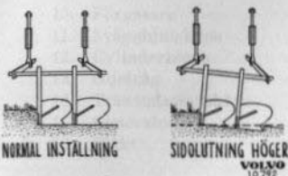
Bild 15. Inställning av hydrauliskt buren plog.
