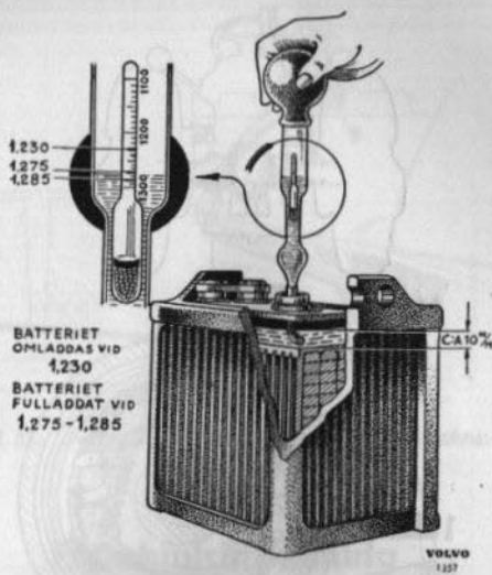
Bild 33. Kontroll av batterielektrolytens specifika vikt och nivå.
