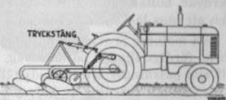
Bild 14. Inställning av hydrauliskt buren plog.
