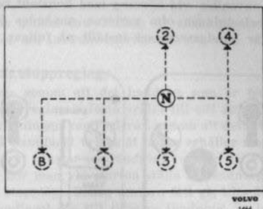
Bild 6. Växelspakens lägen.
