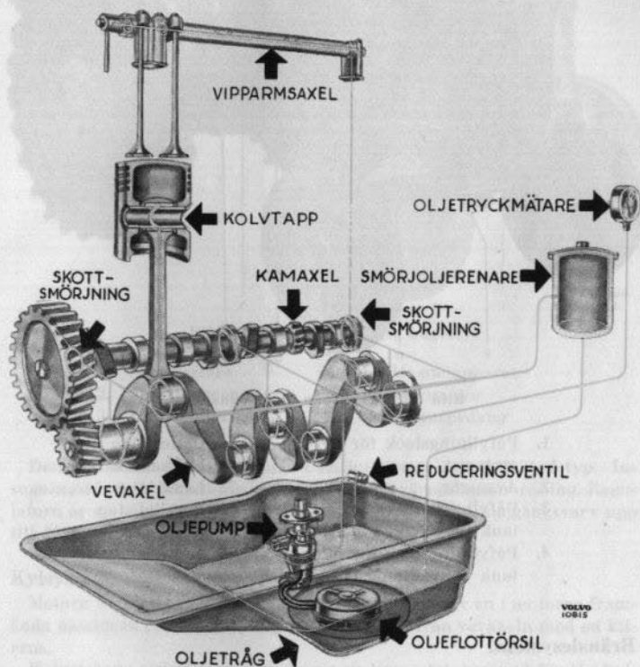
Bild 18. Schematisk framställning av motorns smörjssystem.
