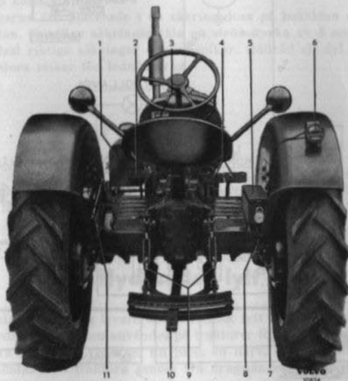
Bild 22. Traktorn bakifrån.
