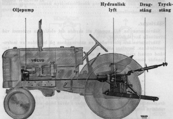
Bild 24. Traktor med hydraulisk lyft.
