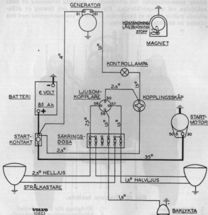
Bild 23. Kopplingsschema för det elektriska systemet.
