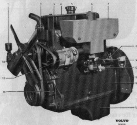
Bild 16. Motorn från vänster.
