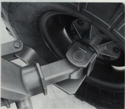
Hydraulisk snedställning av bärhjul. Rekommenderas på fält med svåra sidolut (lagerföres ej).
