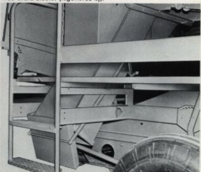
Väldimensionerad stenuppsamlingslåda (standard 644 S, extra utrustning för övriga modeller).
