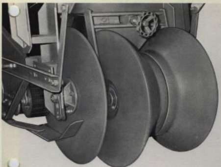
Upptagaraggregatets bärrulle och rullskär som standard utrustade med avskrapare.
