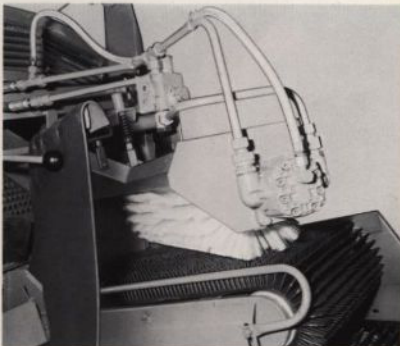
Det hydrauldrivna st enfrånskilningsaggregatet på modell 644 S. Såväl borstens höjd från och vinkel mot gummifingerbandet som hastigheten är inställbara från maskinens plattform.
