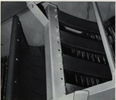
Sällmatta med bromsduk av gummi (standard) samt kokkross, bestående av kraftiga gummistavar (lagerföres ej).
