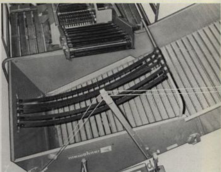
Elevatortank (rymd 2,8 m 3 ) med faldämpande plastband (extra utrustning).
