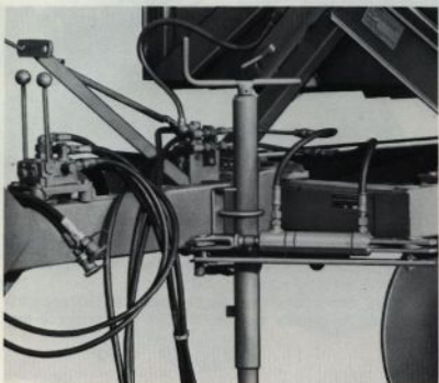
Hydraulisk sidoreglering av draget (extra utrustning).
