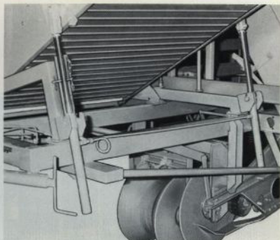
Hydraulreglering av elevatortanken med mekanisk säkerhetsanordning vid servicearbeten under tanken.
