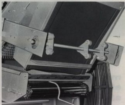
Skakaggregat för montering på modell 644. Lämpligt för starkt kokbildande jordar. Extra utrustning.
