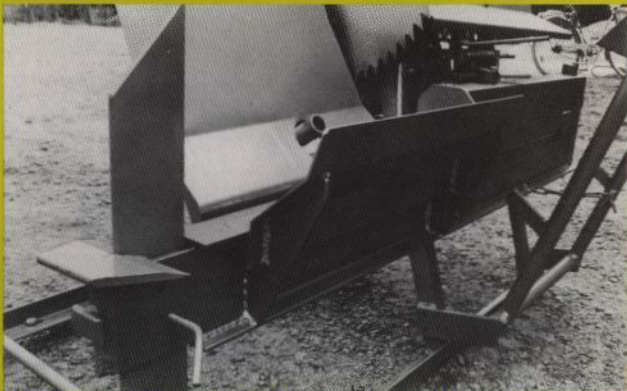
JAPA har en stadig klyvränna, som är också öppen i botten så att spill faller till marken.
