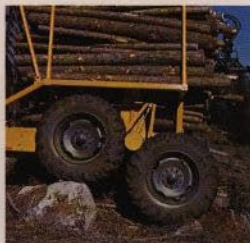
Boggin ger maskinen en förnämlig klätterförmåga och full markkontakt även i mycket kuperad terräng.
