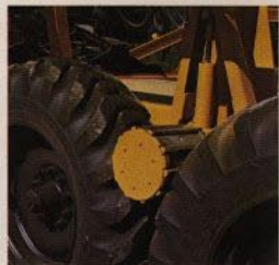
Drivningen av boggin sker från kraftuttaget via en vinkelväxel och drivrullar – en enkel och pålitlig kraftöverföring.
